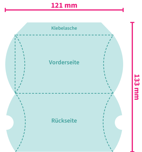
Ihr fertiges Druckprodukt (gestanzt, hier ungefalzt dargestellt – gefalzt 100 x 20 x 60 mm)
